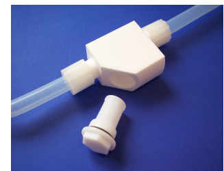
Herausnehmbarer Filterkorb
